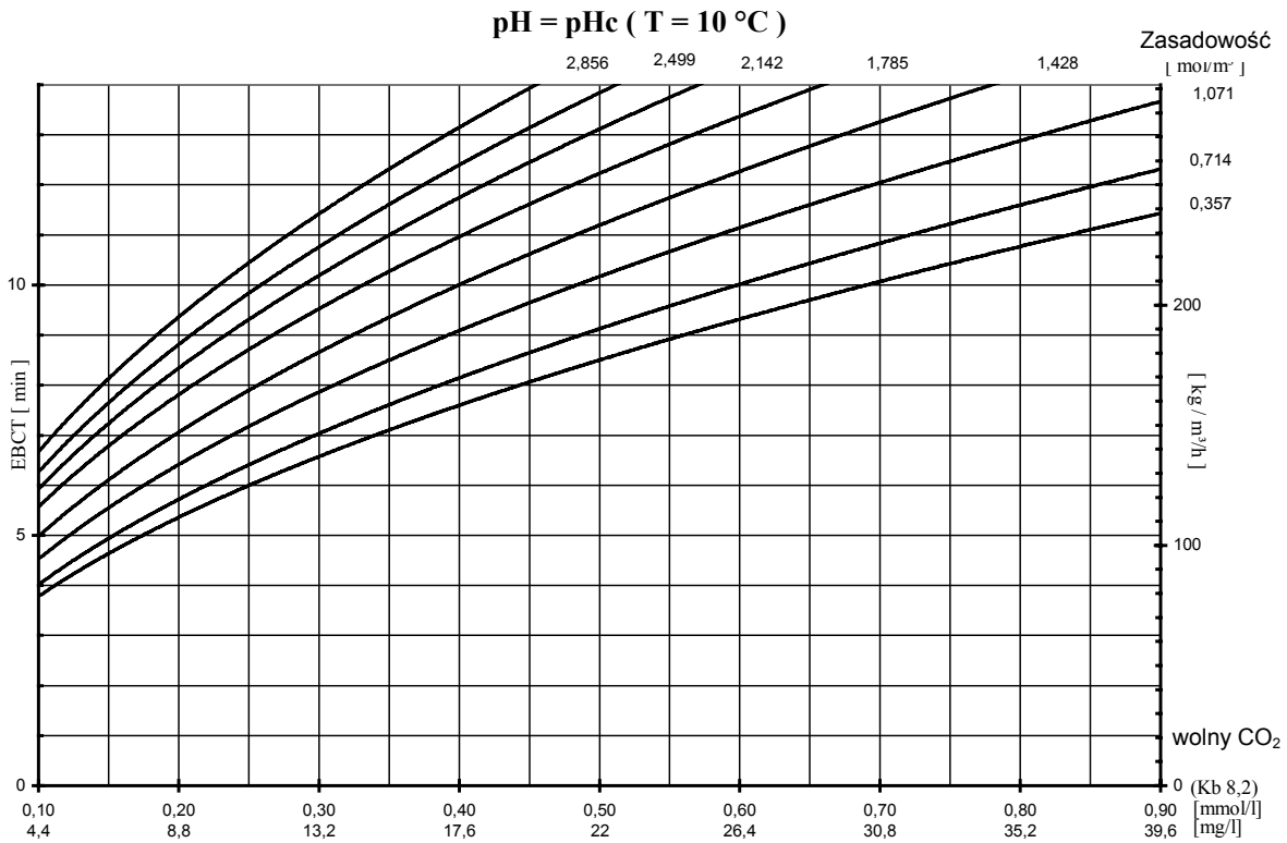
Czas kontaktu EBCT dla złoża AKDOLIT-GRAN, rozmiar I
